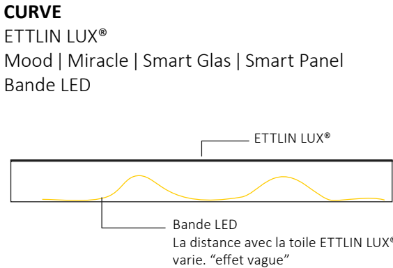
Calpinage LED derrière la toile ETTLIN LUX® Distance de 10 à 20 cm environ
