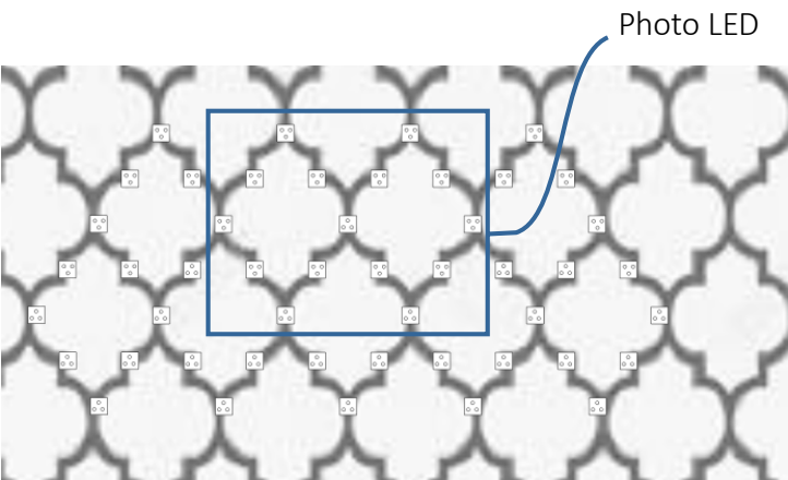
Calpinage LED derrière la toile ETTLIN LUX® Distance de 5 à 20 cm environ
