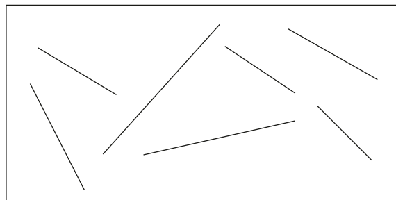
Calpinage LED derrière la toile ETTLIN LUX® Distance de 15 à 25 cm environ
