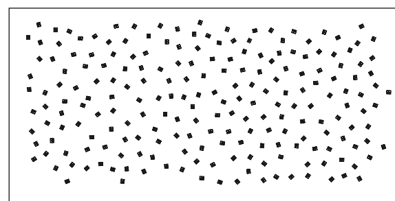
Calpinage LED derrière la toile ETTLIN LUX® Distance de 5 à 20 cm environ
